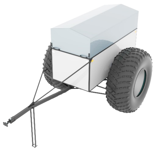
Прицеп одноосный «Бурлак»
